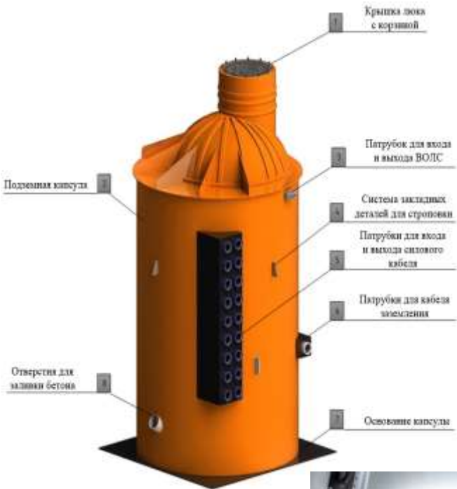
Капсула в сборе
