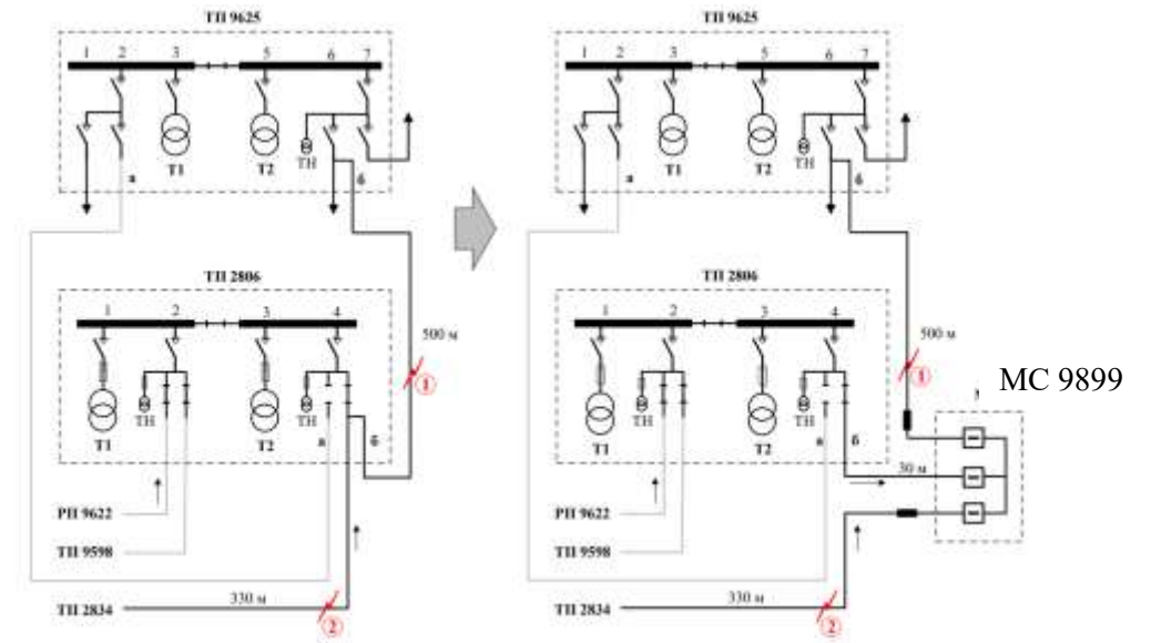
Схема включения MC
